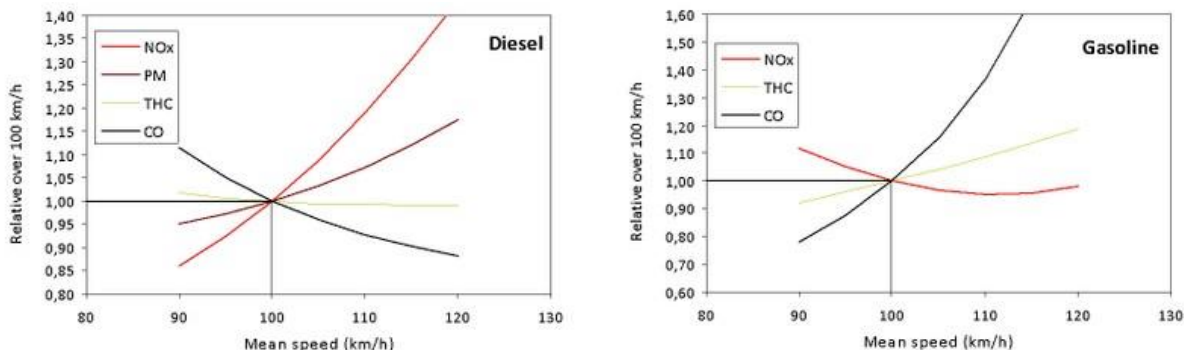
Obr. 44: Závislost produkce emisí škodlivin dieselového motoru (vlevo) a benzínového motoru (vpravo) na rychlosti. (Zdroj EMISIA - ETC/ACM)
