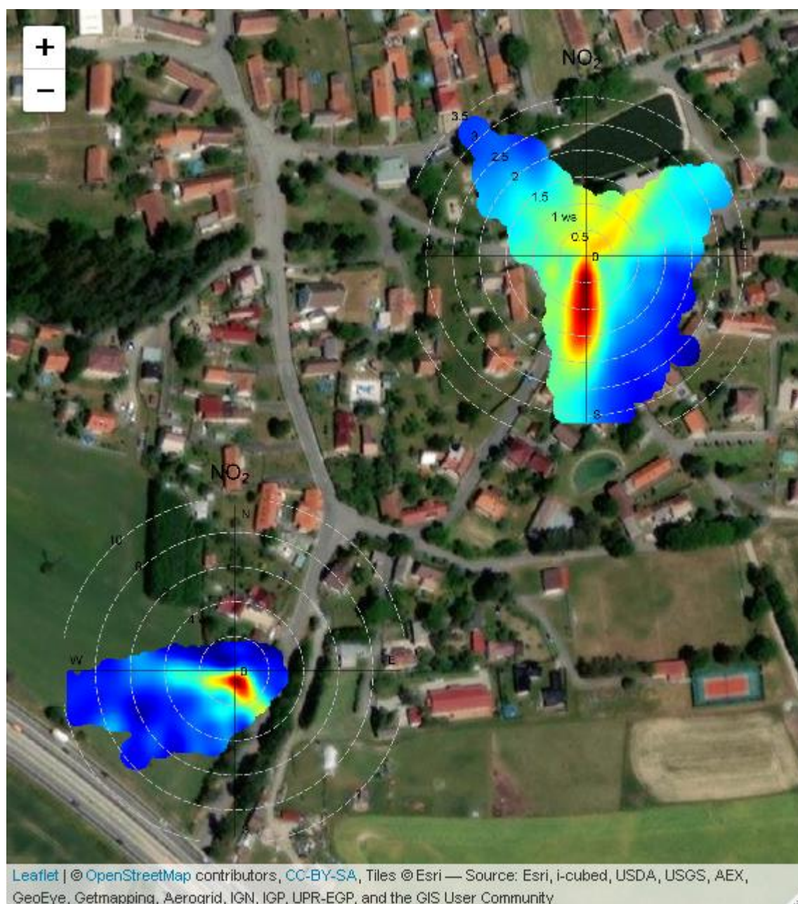
Obr. 42: Koncentrační růžice pro \text{NO}_2 na obou lokalitách (zobrazení koncentrací metodou NWR)
