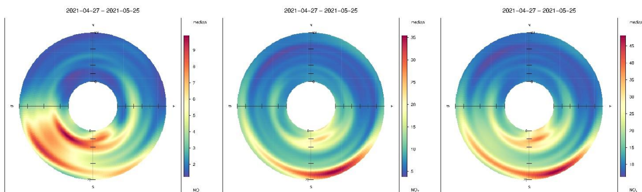
Obr. 39: Denní chod koncentrací NO (vlevo), \text{NO}_2 (uprostřed) a \text{NO}_x (vpravo), lokalita Hulice
