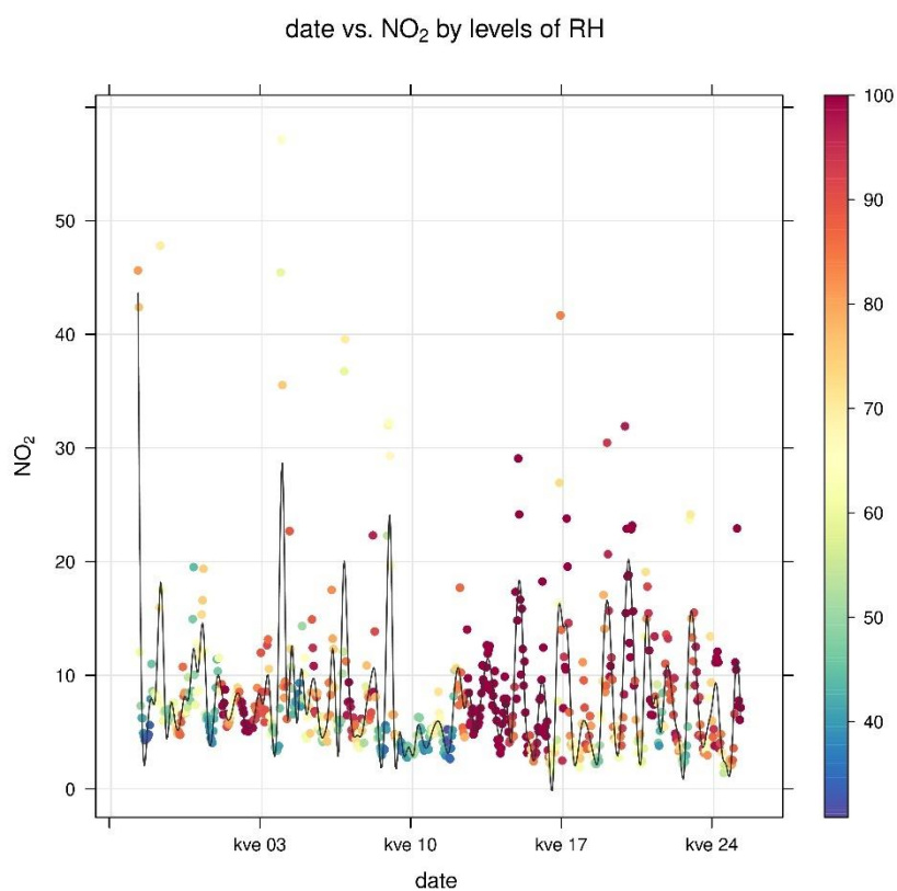
Obr. 36: Průměrné hodinové koncentrace NO 2 v závislosti na relativní vlhkosti vzduchu, lokality Hulice (nahore) a OU Hulice (dole)
