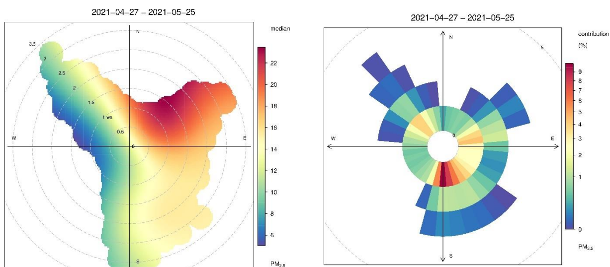
Obr. 25: Koncentrační růžice (vlevo) a vážená koncentrační růžice (vpravo) pro PM_{2,5} , lokalita OU Hulice
