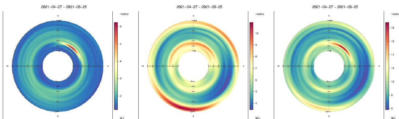
Obr. 40: Denní chod koncentrací NO (vlevo), \text{NO}_2 (uprostřed) a \text{NO}_x (vpravo), lokalita OU Hulice
