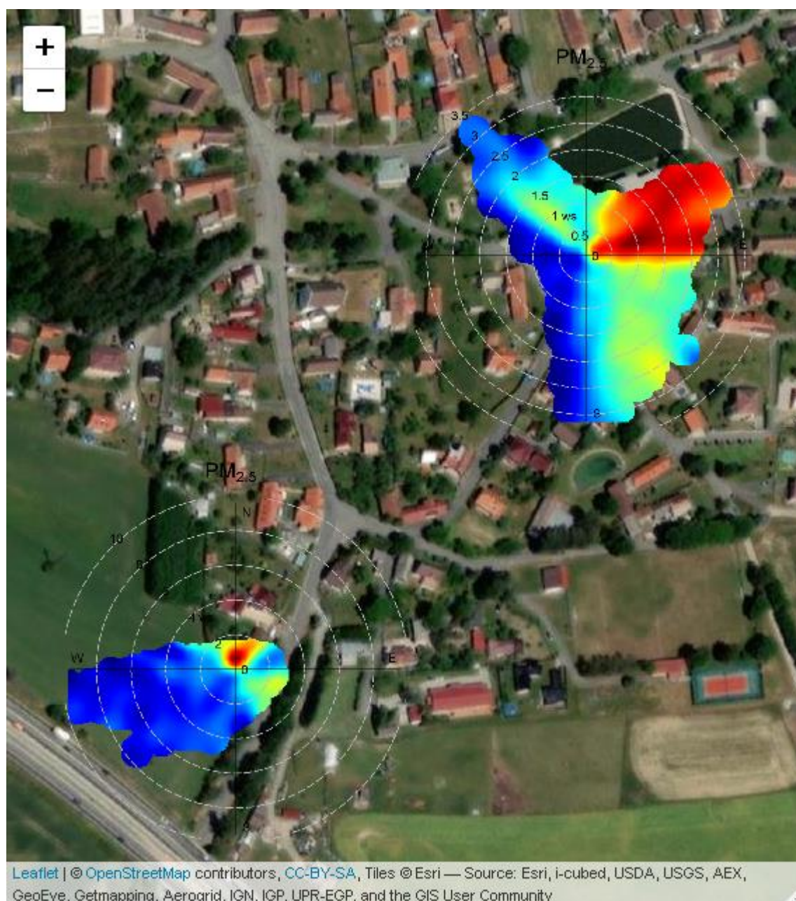
Obr. 30: Koncentrační růžice pro PM 2.5 na obou lokalitách (zobrazení koncentrací metodou NWR)
