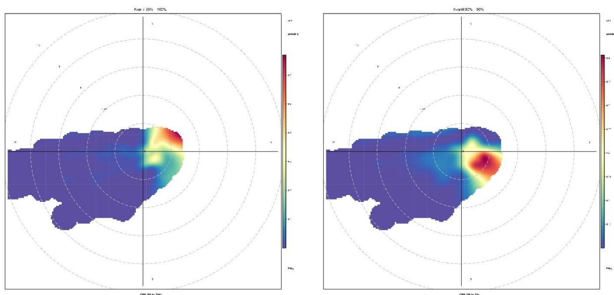
Obr. 19: Pravděpodobnost, při jakých rychlostech a směrech větru je měřeno 10 % nejvyšších minutových koncentrací PM_{10} (vlevo) a druhých 10 % nejvyšších koncentrací PM_{10} (vpravo) na lokalitě Hulice
